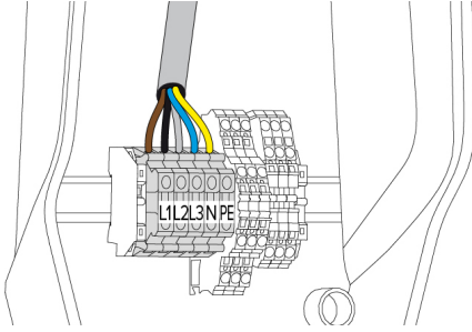
Kuva 8: Jännitesyötön liitanta
