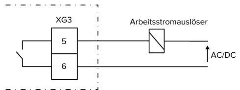
Abb. 9: Prinzipschaltbild: Anschluss eines externen Arbeitsstromauslösers
