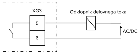
sl. 9: Osnovna vezalna shema: priključitev zunanjega odklopnika delovnega toka
