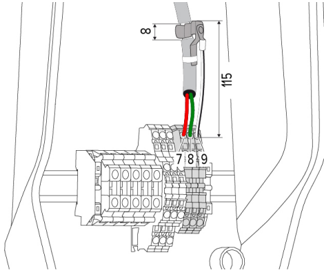
Fig. 10: Ligação da linha de dados [mm]
