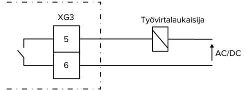
Kuva 9: Periaatekytkentäkaavio: ulkoisen työvirran laukaisijan liitanta
