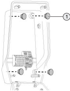
Fig. 7 : Bouchons de fermeture
