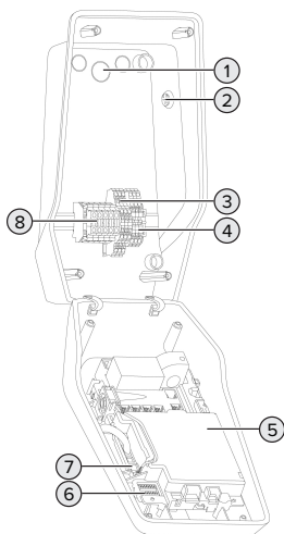
Obr. 4: Pohled dovnitř
