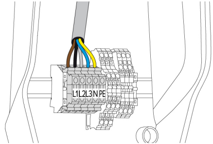
řek. 8: Gerilim beslemesi baęlantısı
