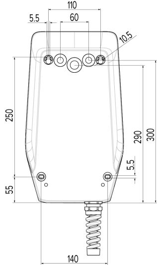
Kuva 6: Porausmitat [mm]
