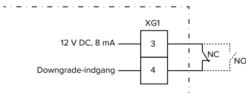
Fig. 13: Principskema: tilslutning af en ekstern omskifterkontakt (standardindstilling: NC)
